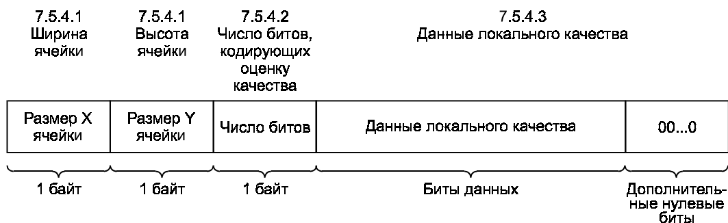
Рисунок 9 — Диаграмма формата данных локального качества
