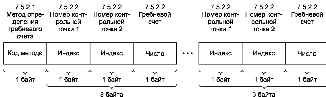
Рисунок 7 — Диаграмма формата данных гребневого счета
