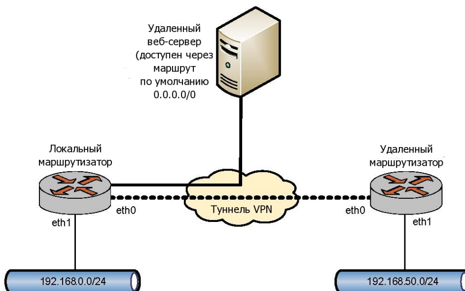
Рисунок 48 - Маскировка и VPN
