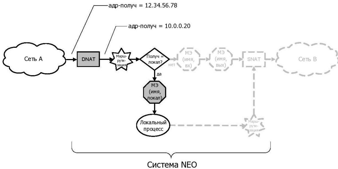
Рисунок 36 - Решения МЭ при использовании DNAT для пакетов, предназначенных системе Altell NEO
