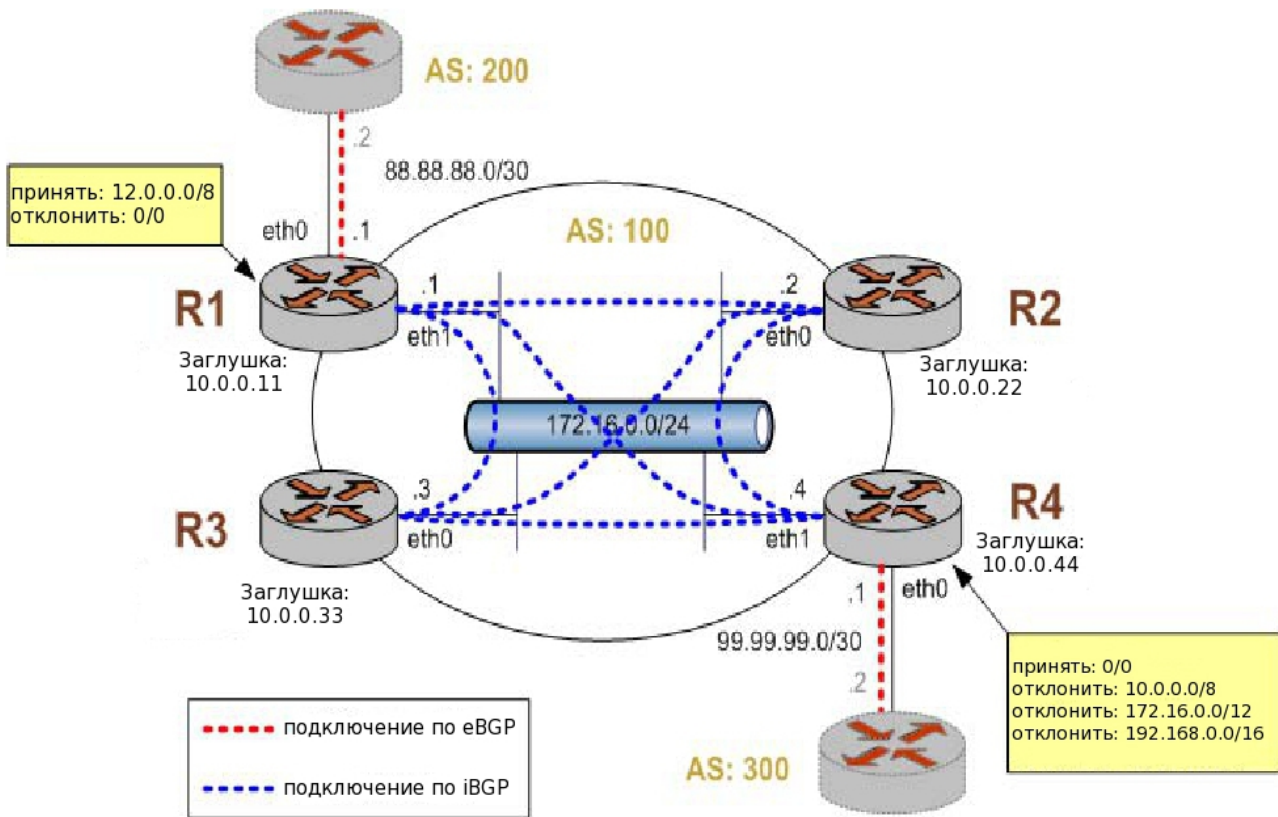
Рисунок 19 - Фильтрация входящих маршрутов
