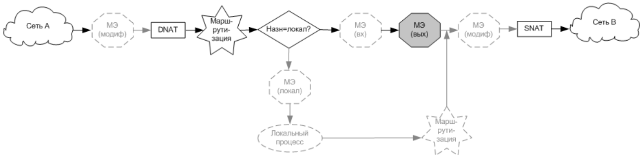
Рисунок 51 - Применение правил фильтрации к транзитному трафику, отправляемому через интерфейс
