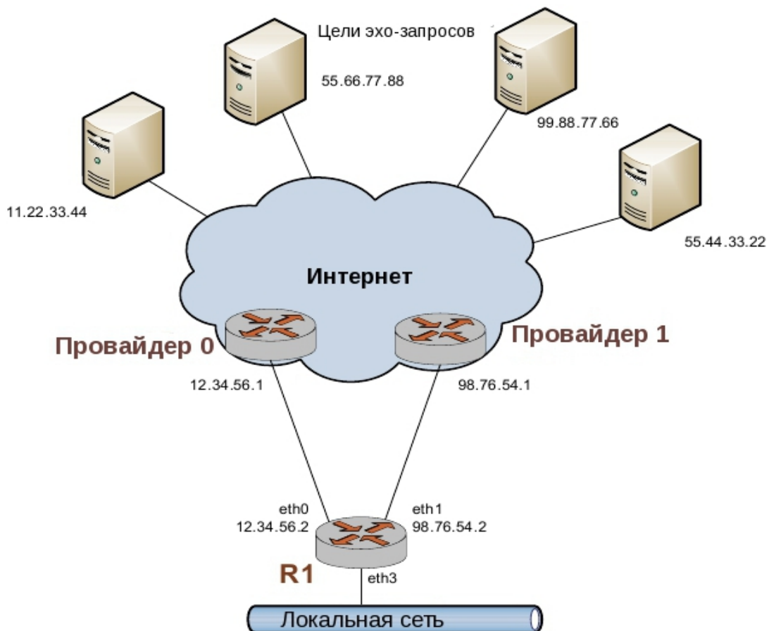
Рисунок 93 - Балансировка нагрузки ГВС
