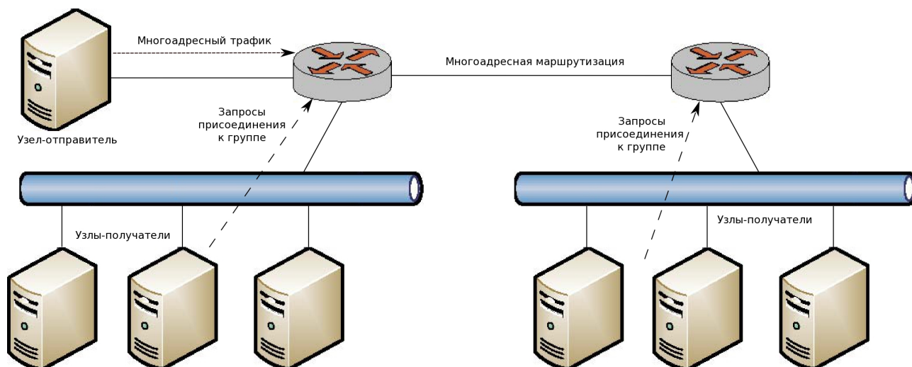
Рисунок 21 - Интрасеть с поддержкой многоадресной передач
