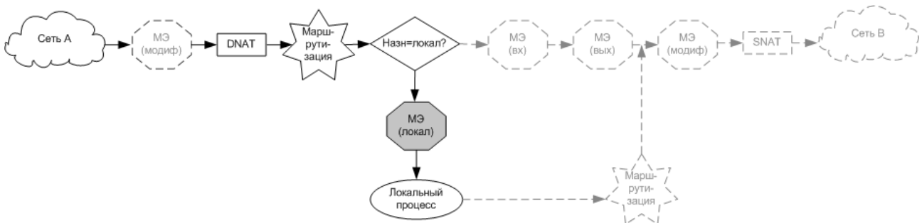
Рисунок 52 - Применение правил фильтрации к трафику, предназначенному локальной системе, получаемому на интерфейсе
