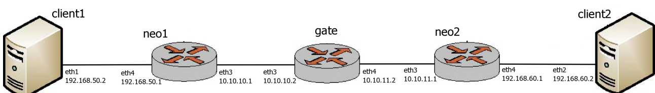
Рисунок 23 - Пример настройки протокола DVMRP с использованием туннелей
