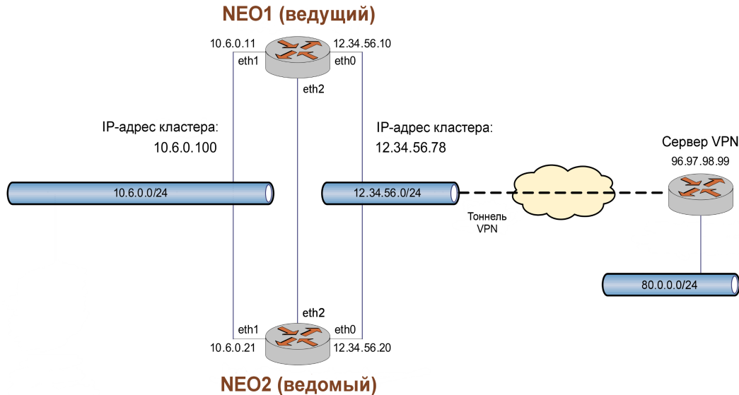
Рисунок 97 - Схема включения кластера как отказоустойчивого клиента VPN
