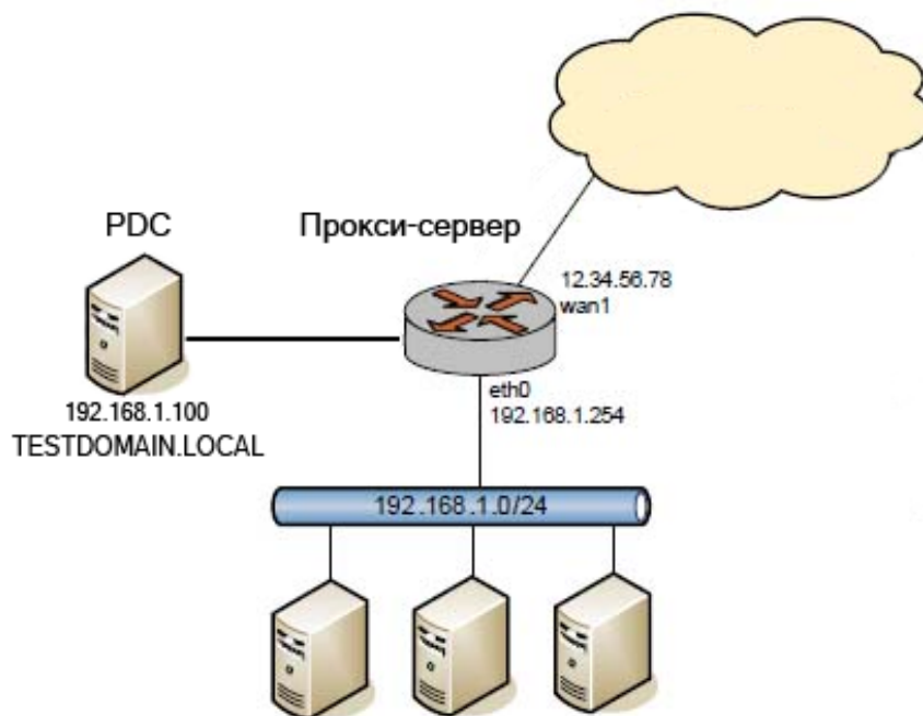
Рисунок 102 - Аутентификация пользователей прокси на основе протокола NTLM
