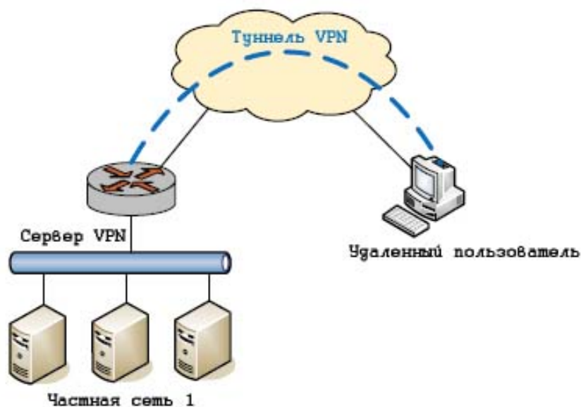
Рисунок 63 - VPN удаленного доступа
