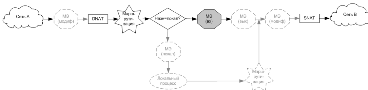
Рисунок 50 - Применение правил фильтрации к транзитному трафику, получаемому на интерфейсе
