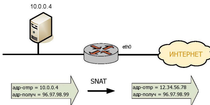
Рисунок 39 - Настройка SNAT (один к одному)
