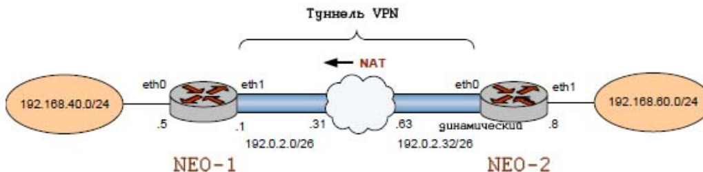
Рисунок 70 - Создание подключения VPN с использованием NAT
