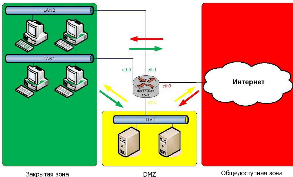
Рисунок 59 - Настройка межсетевого экрана на основе зон безопасности
