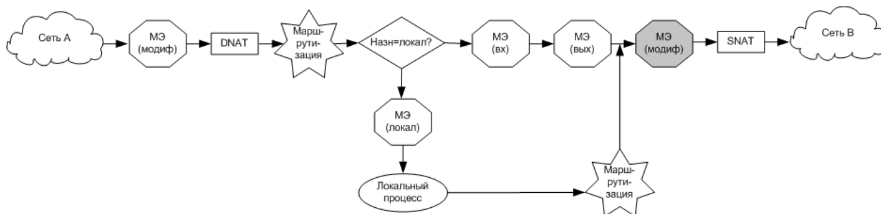
Рисунок 55 - Применение модифицирующих правил к трафику, покидающему интерфейс
