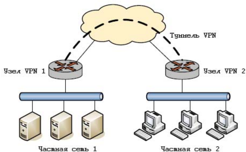
Рисунок 73 - Межфилиальный режим VPN
