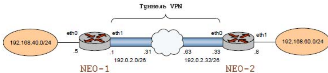
Рисунок 69 - Первичная настройка IPSec в межфилиальном режиме
