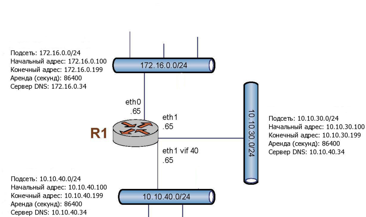
Рисунок 87 - Настройка пулов адресов
