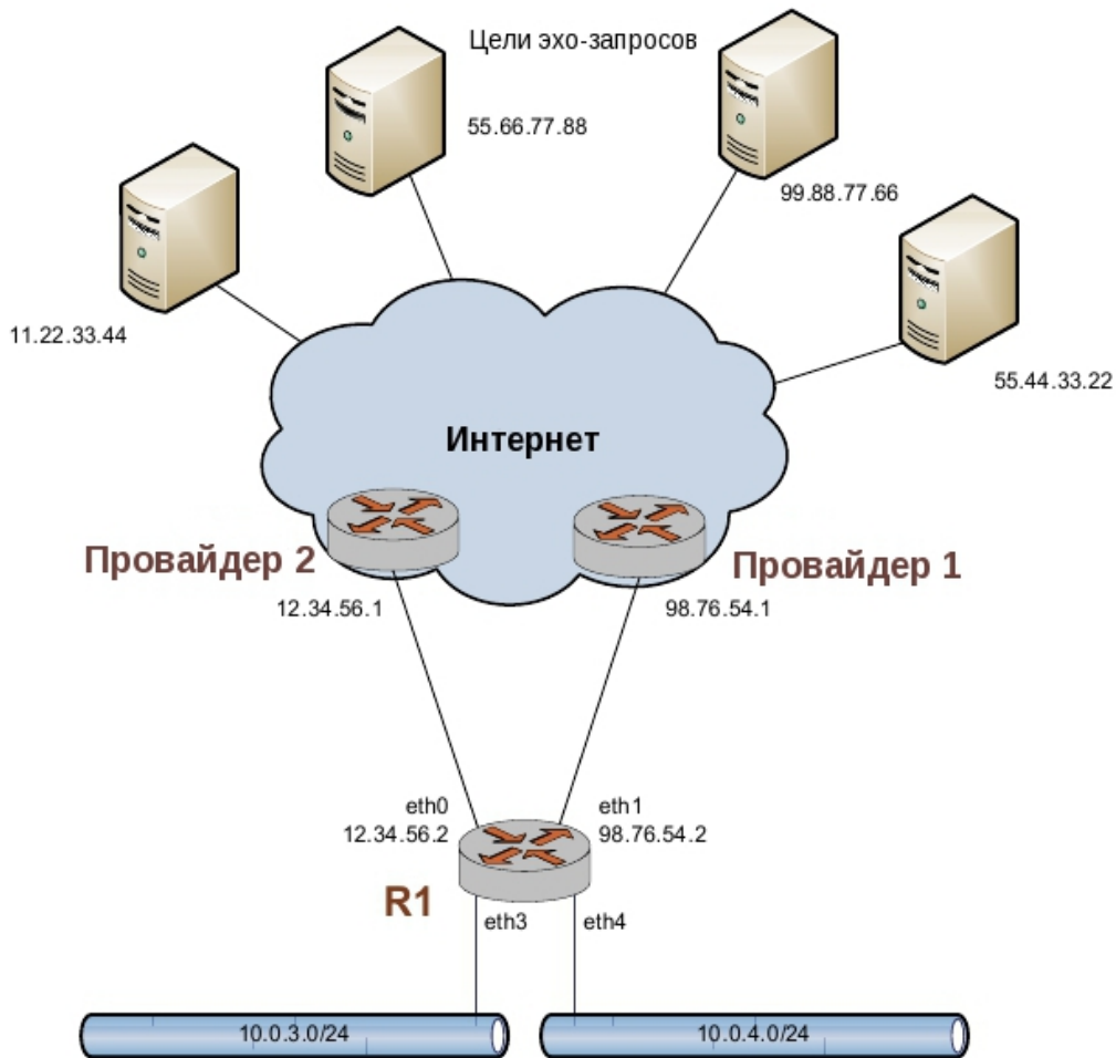
Рисунок 94 - Балансировка нагрузки ГВС при двух локальных сетях
