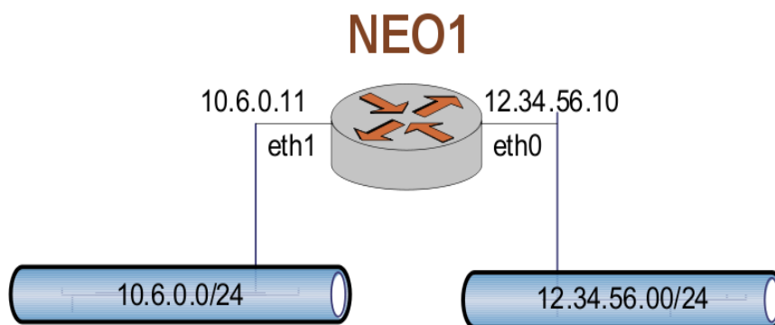
Рисунок 95 - Обычное подключение маршрутизатора
