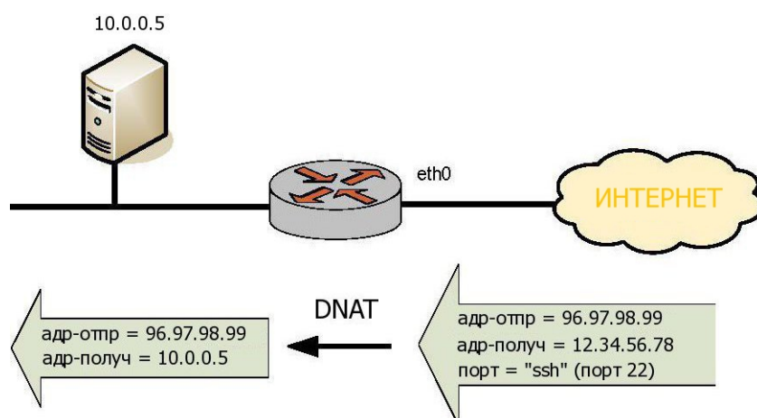
Рисунок 45 - Настройка DNAT (один к одному) - фильтрация по имени порта
