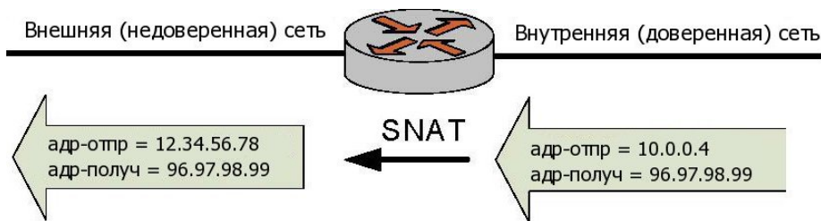
Рисунок 27 - Преобразование сетевого адреса отправителя (SNAT)
