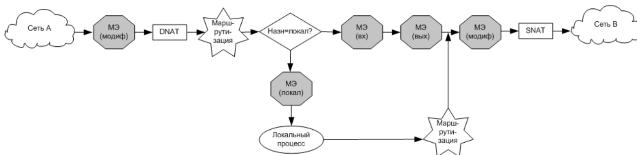
Рисунок 49 - Прохождение трафика через Altell NEO
