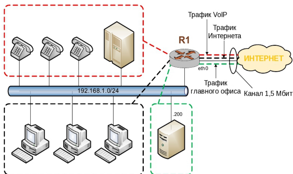
Рисунок 92 - Пример филиала с VoIP с использованием QoS
