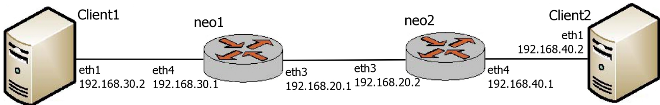
Рисунок 22 - Простейший пример настройки маршрутизации многоадресных передач
