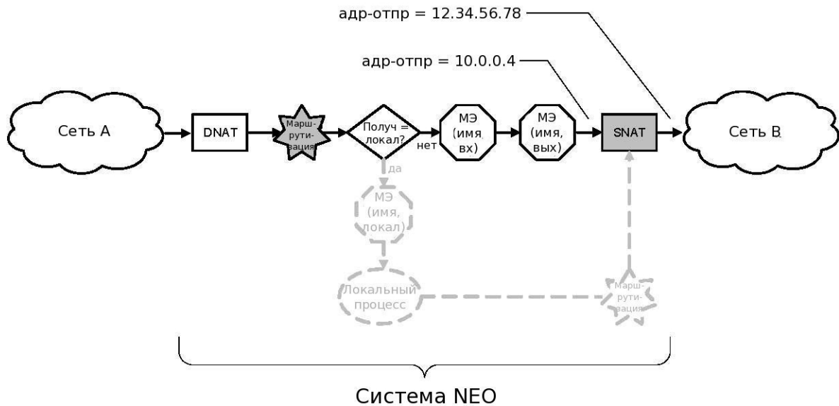
Рисунок 33 - Решения о маршрутизации при прохождении SNAT
