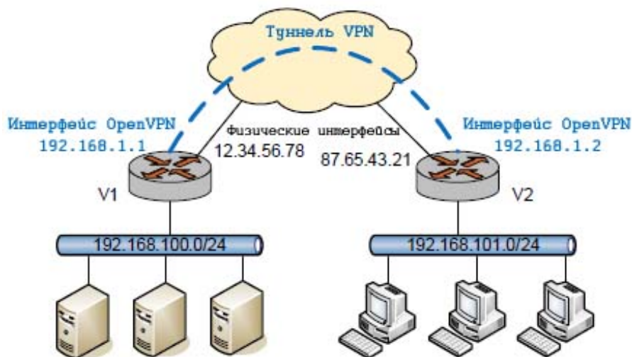
Рисунок 84 - Пример подключения в межфилиальном режиме между узлами V1 и V2 с использованием предварительных ключей
