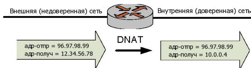
Рисунок 28 - Преобразование сетевых адресов получателя (DNAT)
