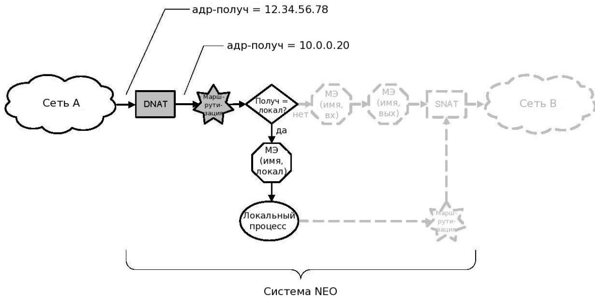
Рисунок 32 - Решения о маршрутизации при использовании DNAT для пакетов, предназначенных системе Altell NEO
