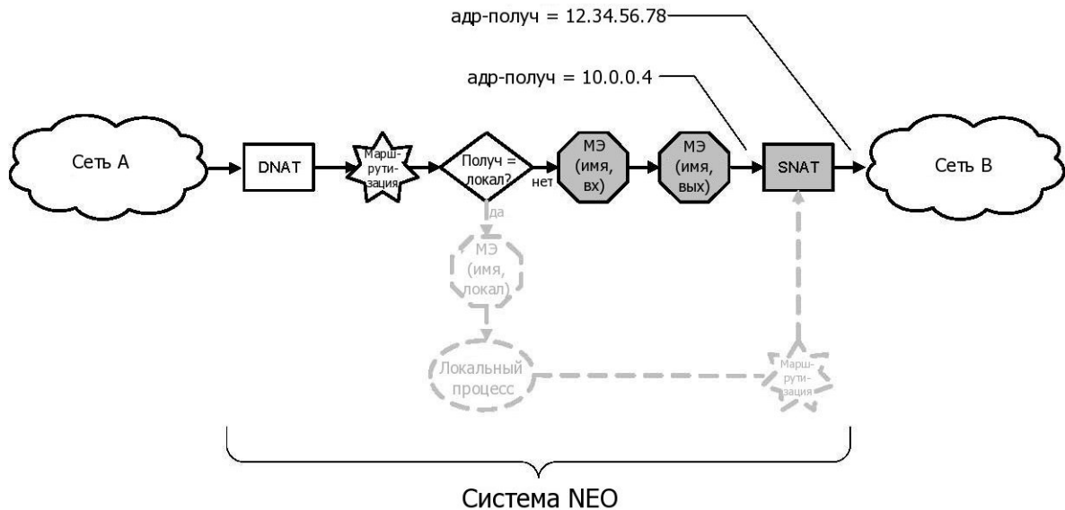
Рисунок 37 - Решения МЭ при использовании SNAT для пакетов, проходящих через систему Altell NEO
