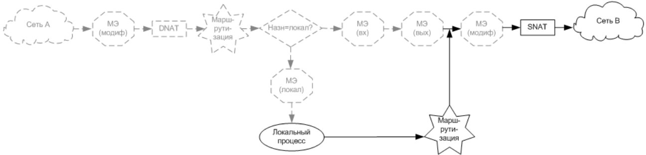
Рисунок 53 - Прохождение трафика, направленного из локальной системы, через Altell NEO
