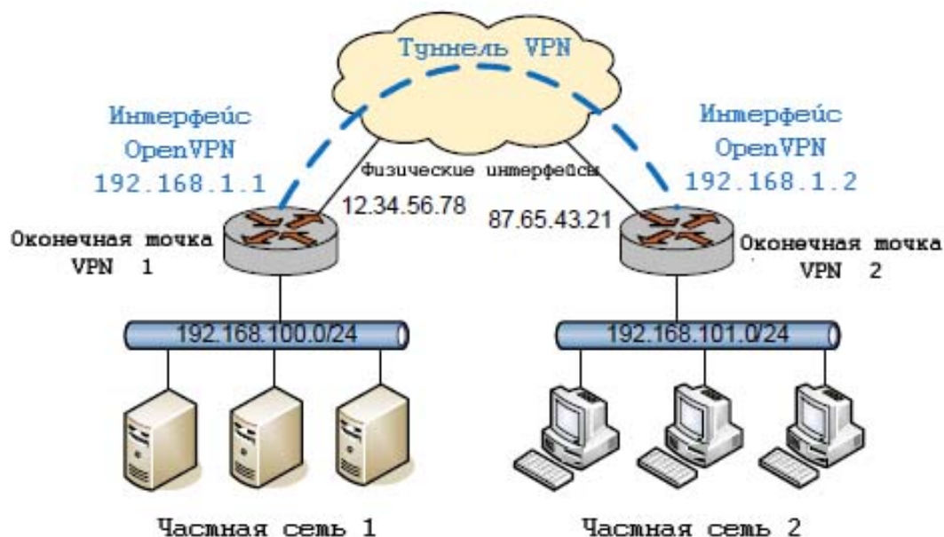
Рисунок 82 - VPN в межфилиальном режиме на базе OpenVPN
