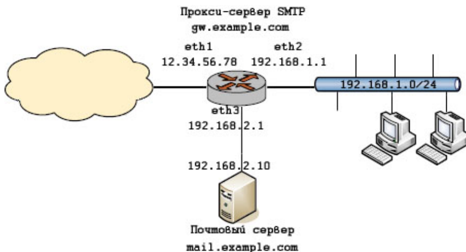
Рисунок 100 - Режим проксирования для заданного сервера
