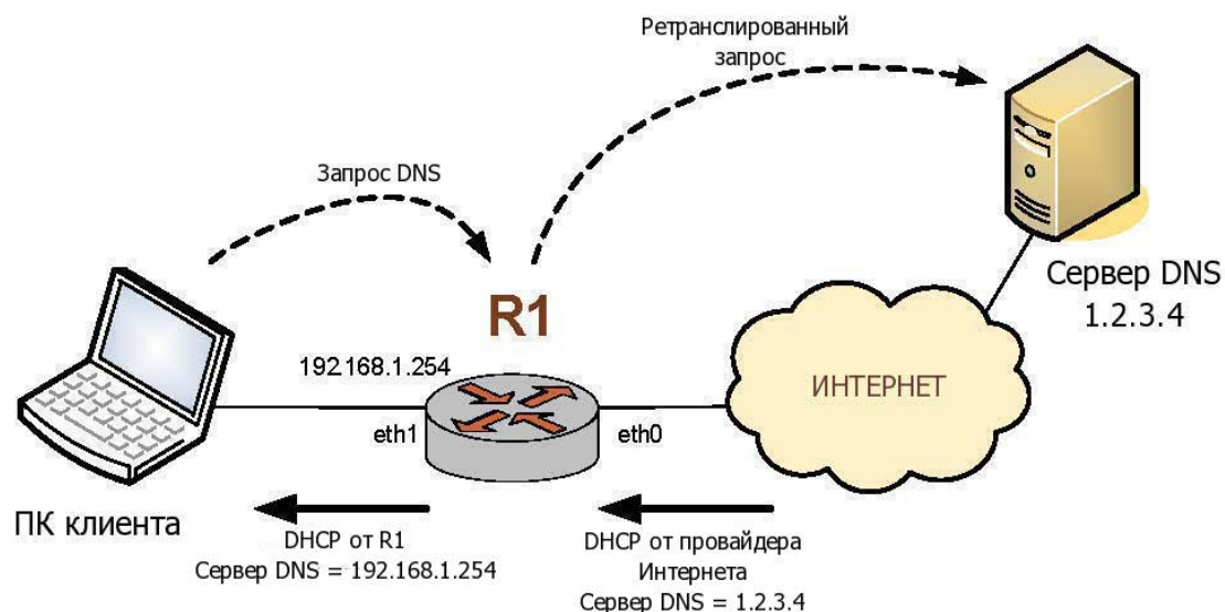
Рисунок 90 - Схема использования ретрансляции DNS
