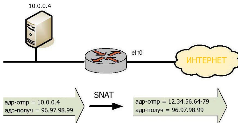
Рисунок 42 - Настройка SNAT (один ко многим)
