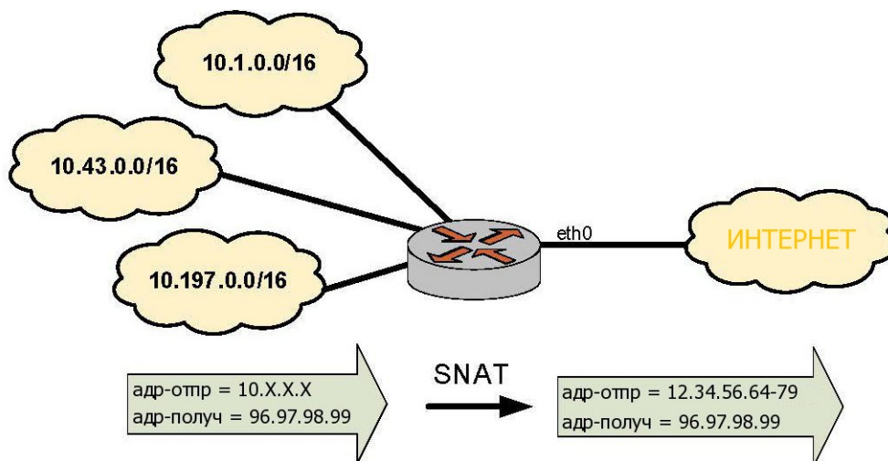
Рисунок 41 - Настройка SNAT (многие ко многим)
