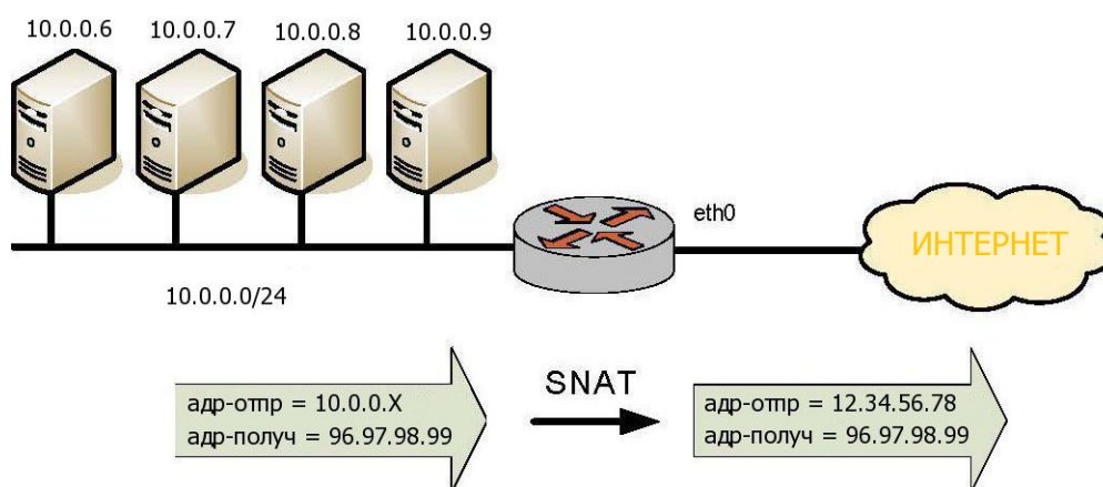
Рисунок 40 - Настройка SNAT (многие к одному)
