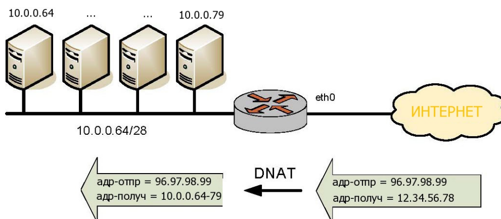
Рисунок 46 - Настройка DNAT (один ко многим)
