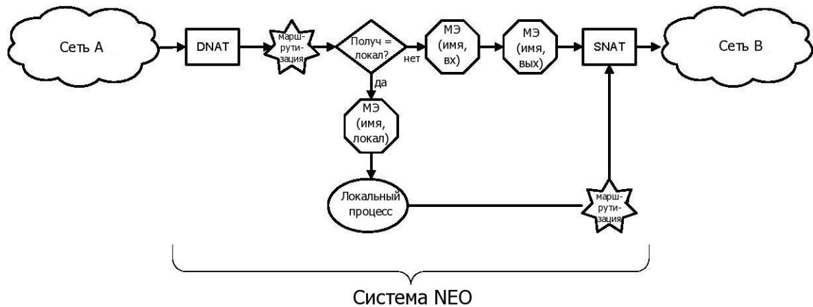
Рисунок 30 - Прохождение трафика через систему Altell NEO
