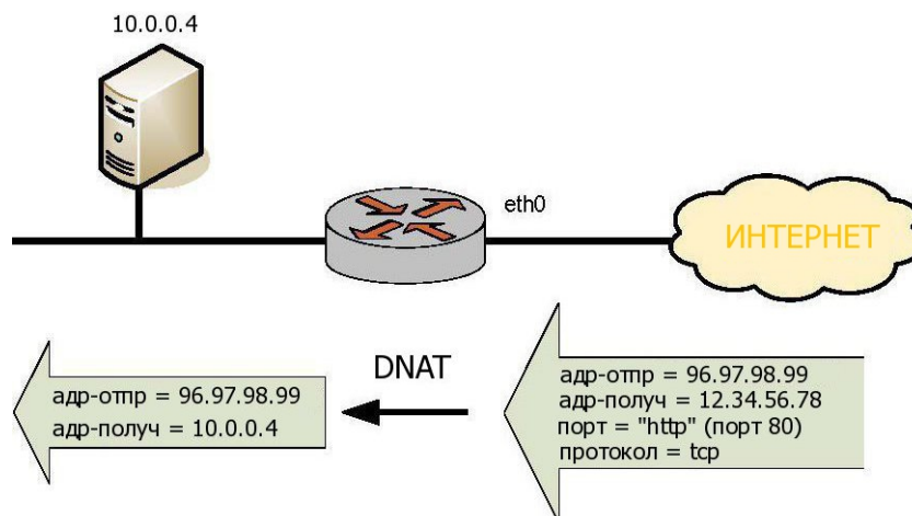
Рисунок 44 - Настройка DNAT (один к одному)
