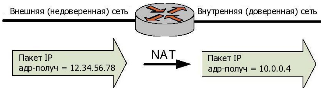
Рисунок 24 - Пример устройства, выполняющего преобразование сетевых адресов (NAT)
