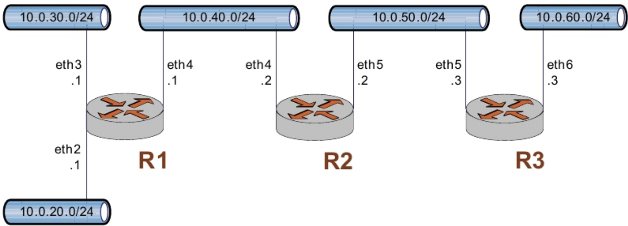
Рисунок 18 - Эталонная схема настройки RIP
