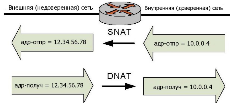
Рисунок 29 - Двухнаправленное преобразование сетевых адресов
