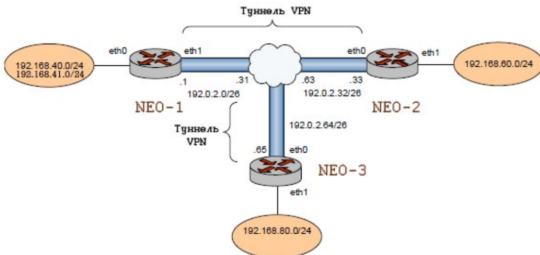
Рисунок 71 - Настройка туннелей IPSec между тремя шлюзами
