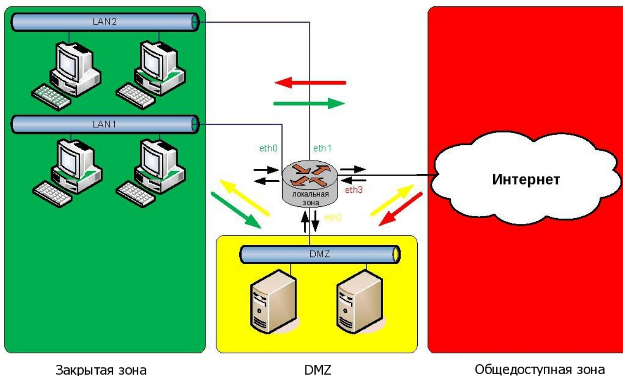
Рисунок 60 - Передача трафика в транзитные зоны и из транзитных зон
