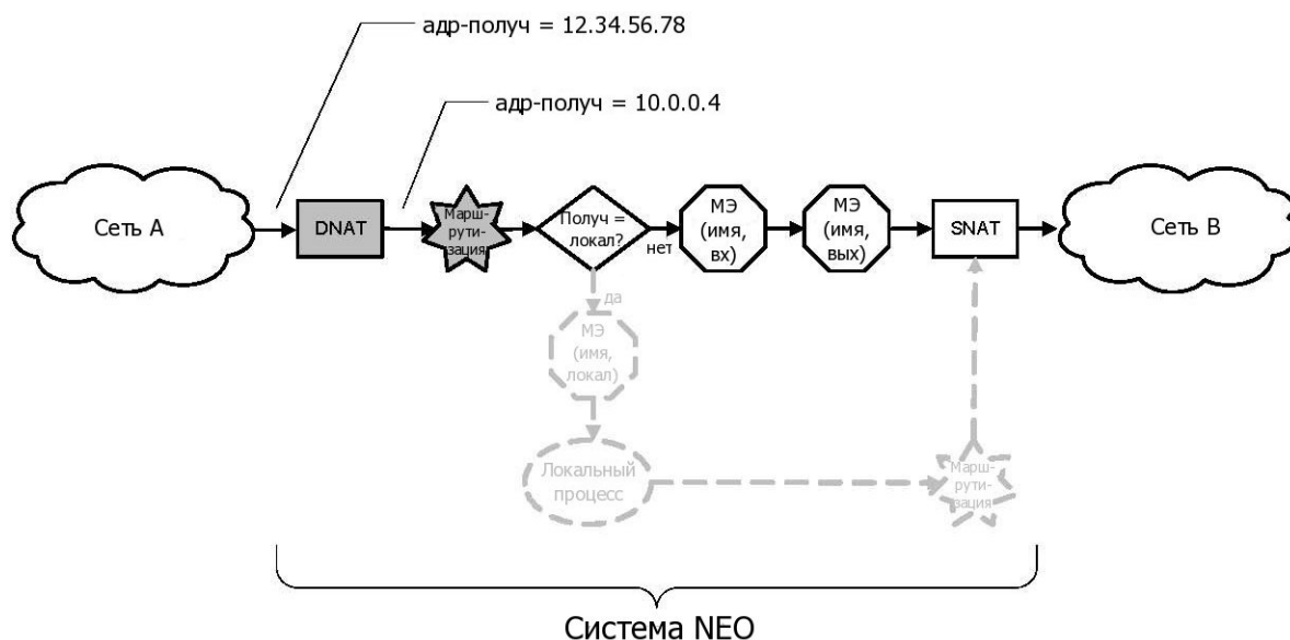
Рисунок 31 - Решения о маршрутизации при прохождении DNAT
