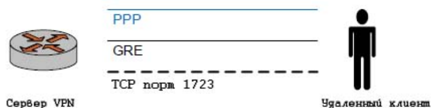
Рисунок 65 - VPN удаленного доступа на основе протокола PPTP
