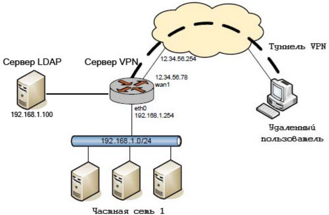
Рисунок 81 - Построение VPN удаленного доступа с аутентификацией на основе LDAP
