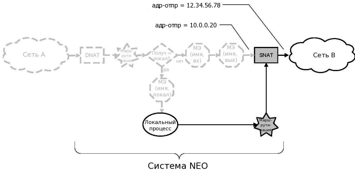
Рисунок 34 - Решения о маршрутизации при использовании SNAT для пакетов, отправленных системой Altell NEO
