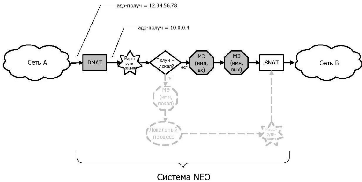
Рисунок 35 - Решение МЭ при прохождении DNAT
