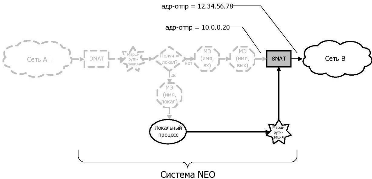
Рисунок 38 - Решения МЭ при использовании SNAT для пакетов, отправленных системой Altell NEO
