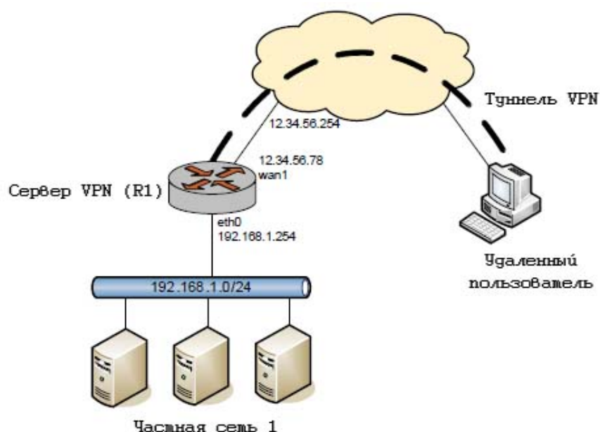
Рисунок 80 - Пример настройки VPN удаленного доступа
