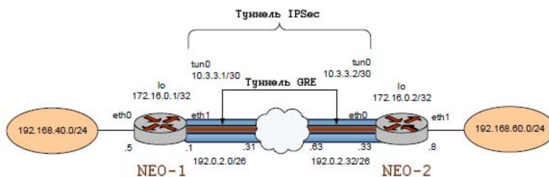
Рисунок 72 - Создание подключения в межфилиальном режиме от узла NEO-1 к узлу NEO-2
