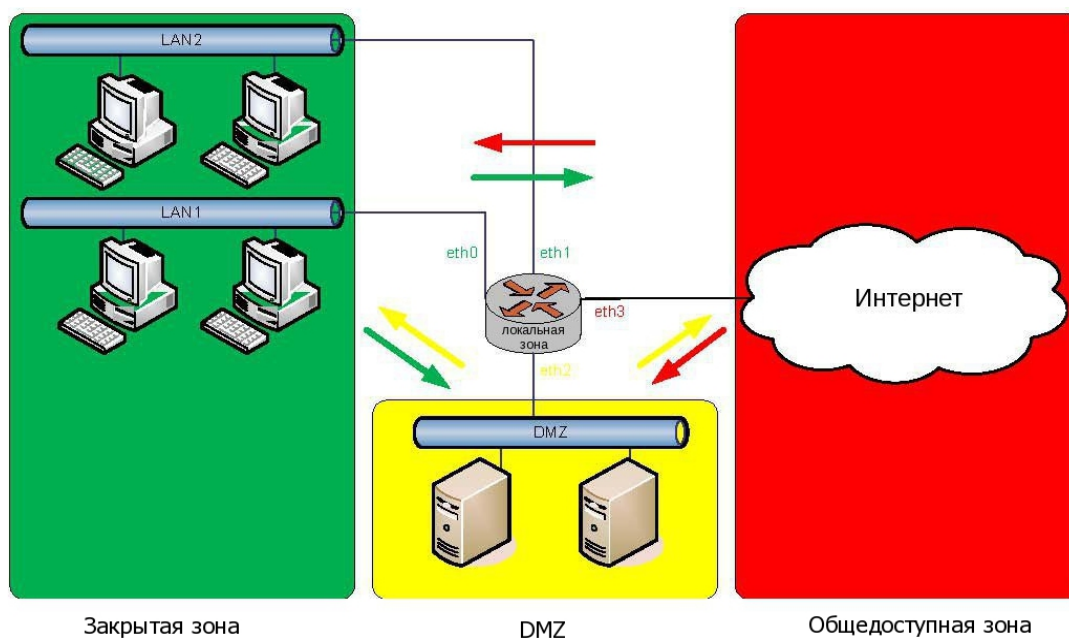
Рисунок 56 - Межсетевой экран, основанный на политиках зон безопасности
